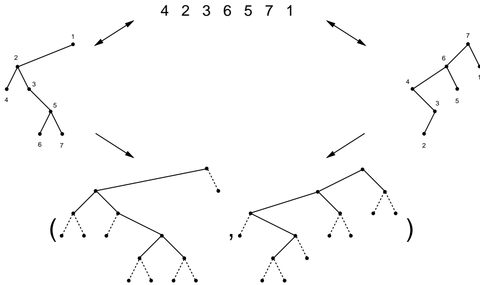
Figure 2: Une permutation de Baxter, ses arbres binaires croissant et décroissant, et les arbres jumeaux lui correspondant.
