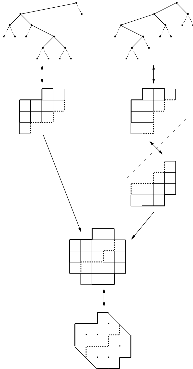
Figure 4: Des arbres jumeaux aux triplets de chemins deux à deux disjoints.
