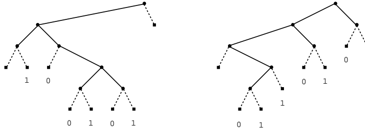
Figure 1: Deux arbres jumeaux de J_7 .
