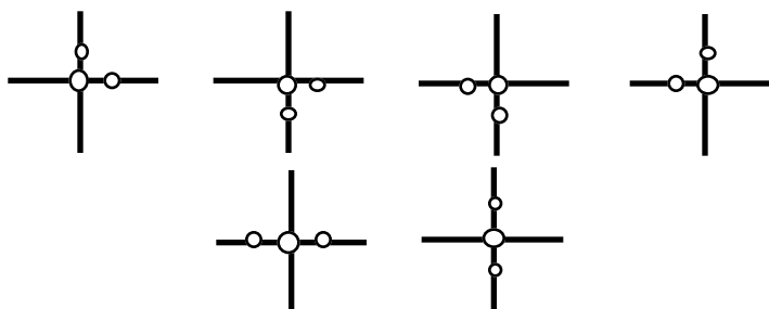
○ : atome d'oxygène ○ : atome d'hydrogène fig. 9
